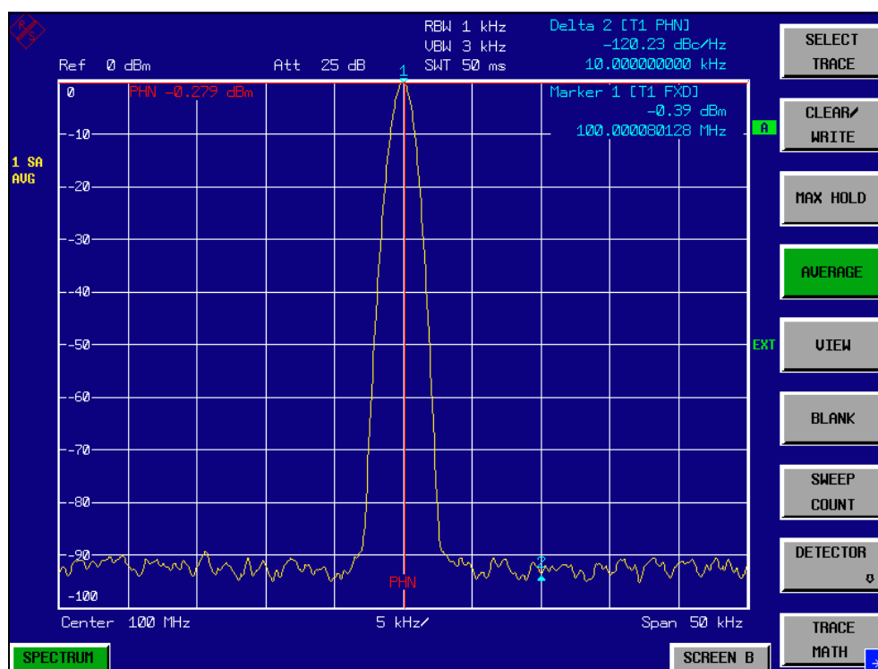
Fig. 2-1 Messung des Phasenrauschens mit der Marker-Funktion Phase Noise
